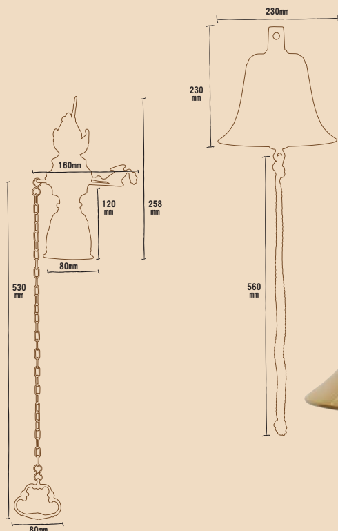
02 シップベル XL 650045
