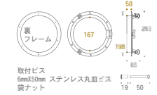
620890 真鍮丸窓 7A 50 C (クローム仕上げ)
