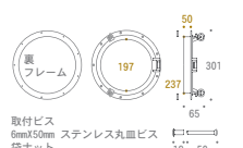
620891 真鍮丸窓 7B 50 C (クローム仕上げ)
