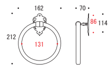
01. タオルリング AR
